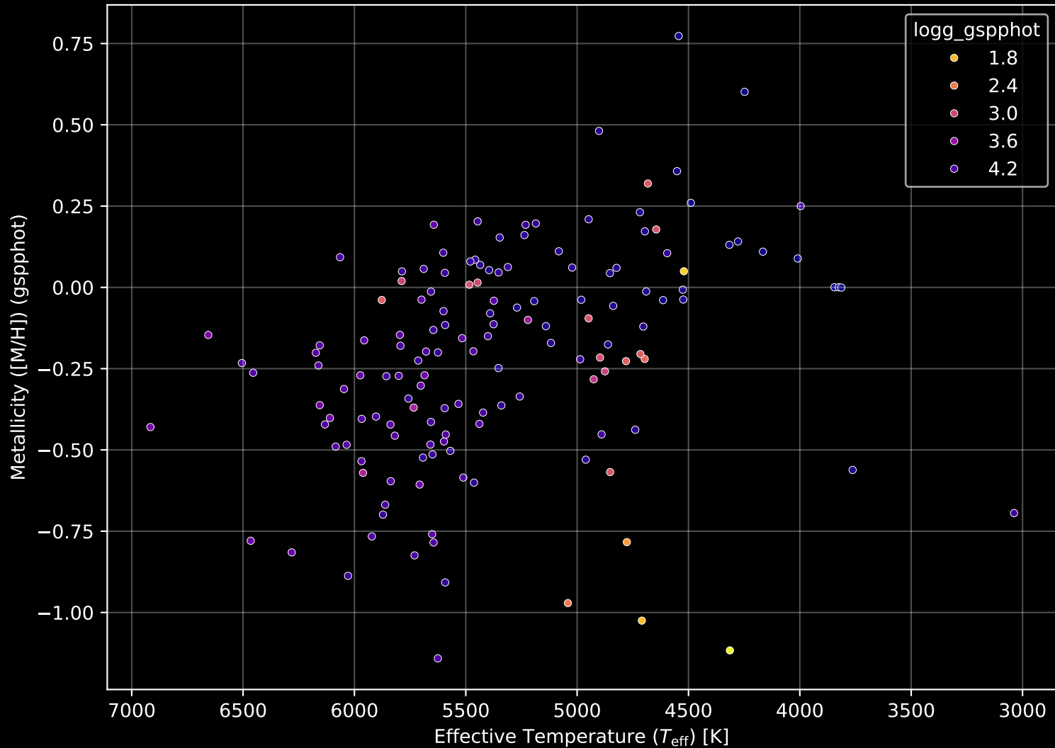
APOGEE DR17 Field: [045+56_MGA] Stellar Population Parameters (n= 148)
